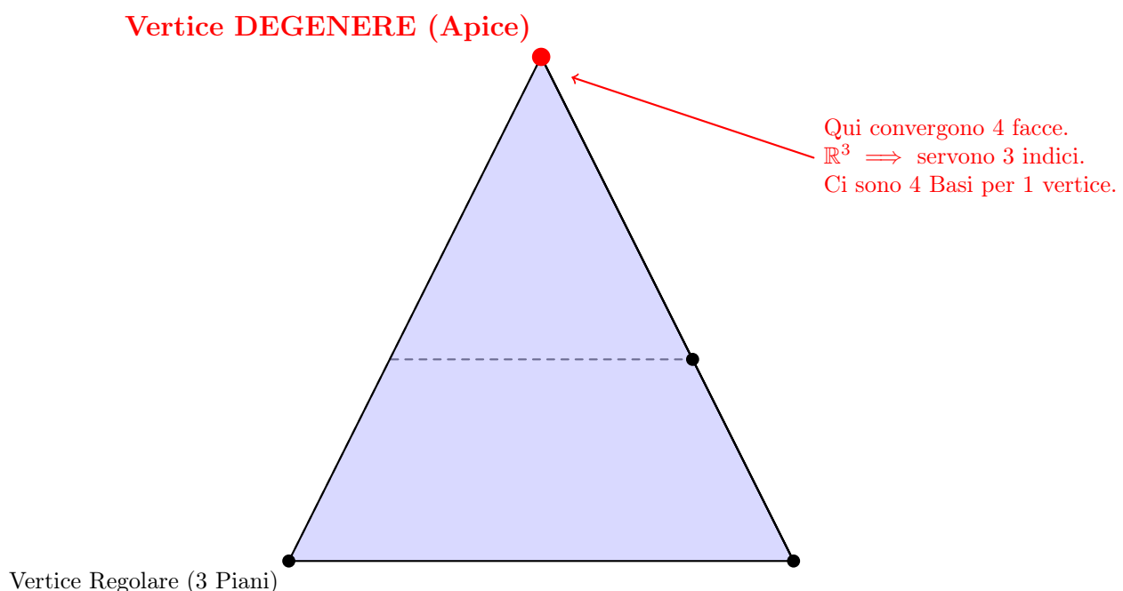
Figura 15. Visualizzazione 3D del concetto di Degenerazione. In un problema a 3 variabili ( n = 3 ), per formare una base occorrono 3 vincoli (piani). Gli angoli della base sono formati esattamente dall'incrocio di 3 piani. L'apice è formato dall'incrocio di 4 piani, superando il numero n . Pertanto è una soluzione degenerare in cui molteplici basi algebriche descrivono lo stesso punto geometrico.
