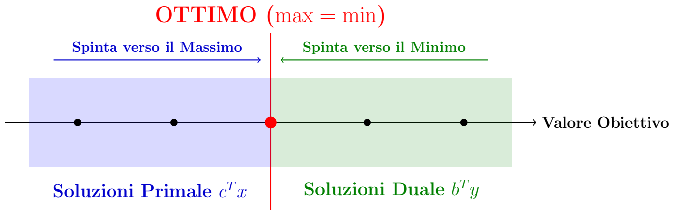
Figura 18. Rappresentazione del Teorema della Dualità Forte. Qualsiasi soluzione primale restituisce un valore inferiore (o al più uguale) a qualsiasi soluzione duale. L'ottimo si verifica nel punto esatto di collisione tra il massimo sforzo del primale e il minimo sforzo del duale.
