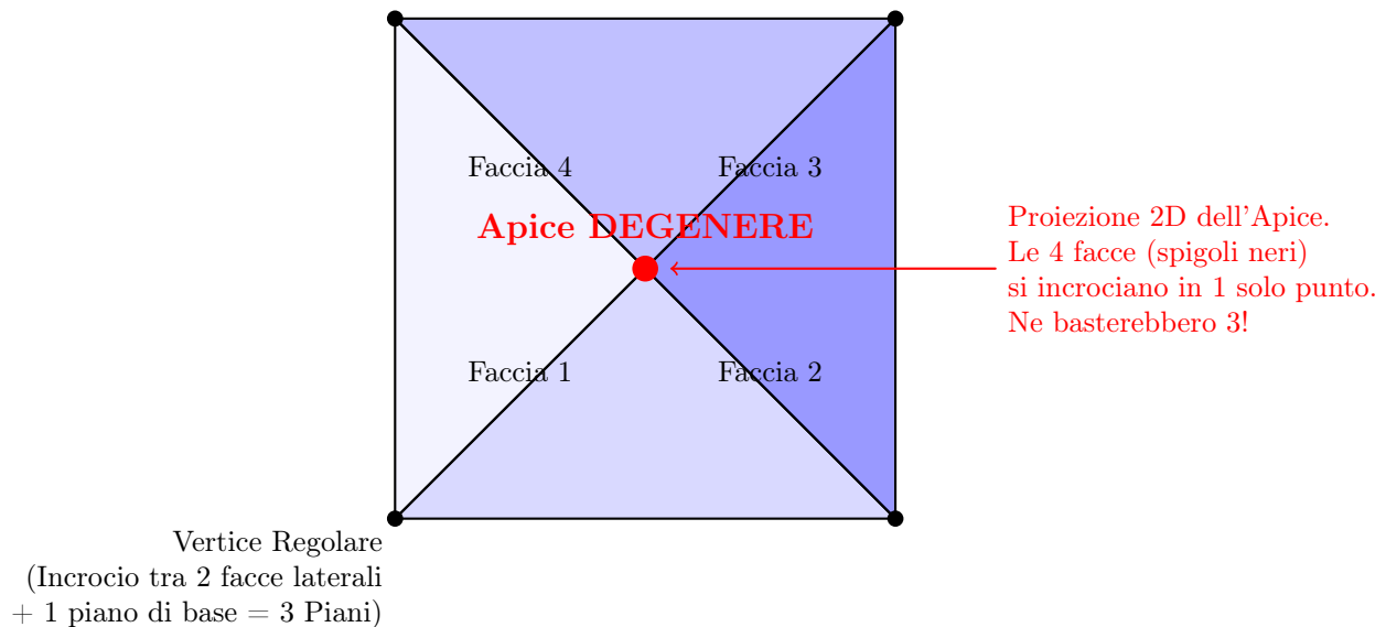
Figura 16. Vista dall'alto (proiezione ortogonale) della piramide. Da questa prospettiva emerge chiaramente l'anomalia matematica della degenerazione: l'apice è il punto di intersezione in cui collidono simultaneamente ben 4 facce (linee nere). Essendo in uno spazio a 3 variabili ( \mathbb{R}^3 ), l'intersezione di 4 piani in un solo punto crea una ridondanza che genera le molteplici basi degeneri.
