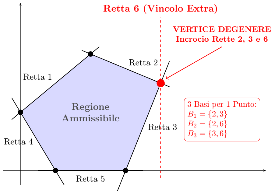
Figura 17. Rappresentazione 2D di un vertice degenera su un pentagono. In uno spazio a 2 variabili occorrono due rette per trovare un vertice. Nel vertice evidenziato in rosso convergono simultaneamente 3 rette (la 2, la 3 e la 6). Questo crea una ridondanza per la quale 3 sistemi lineari differenti (le tre basi B_1, B_2, B_3 ) produrranno matematicamente le stesse coordinate geometriche.
